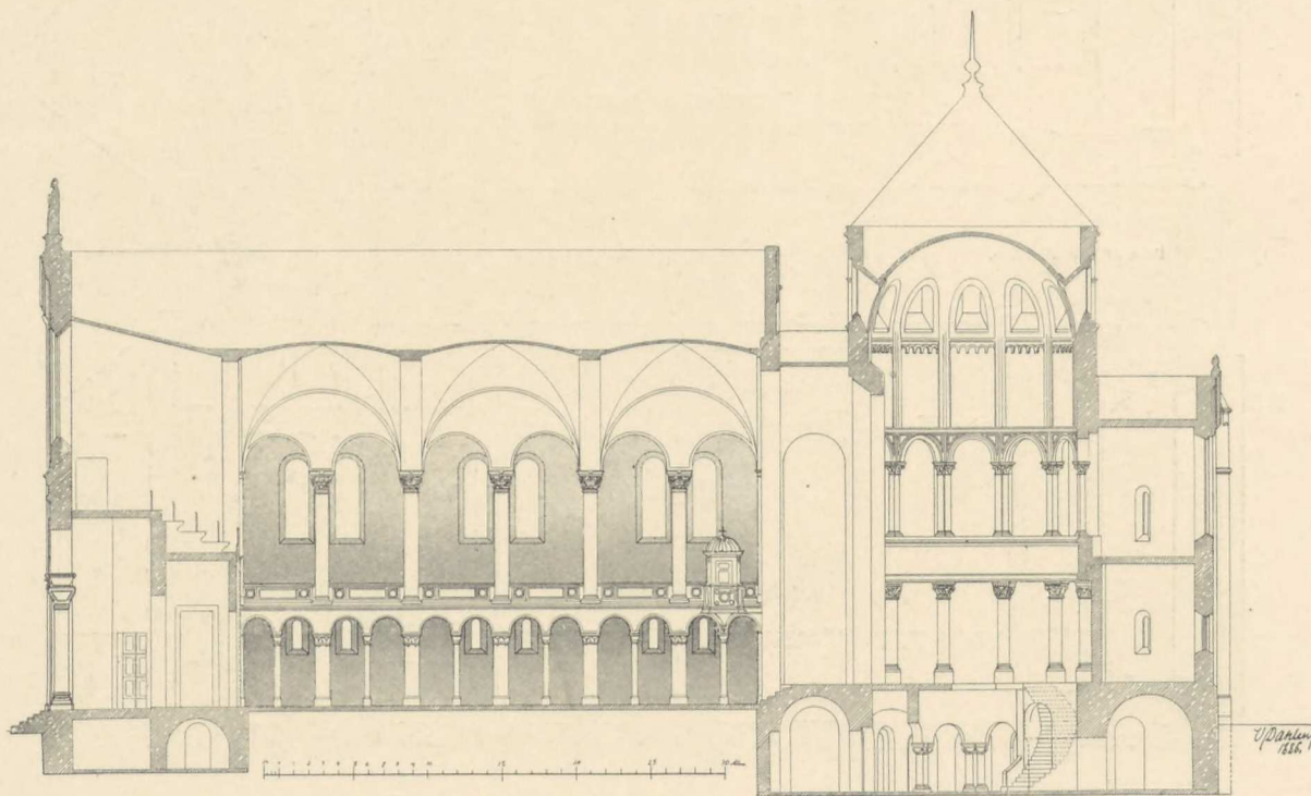
Længdesnit af Jesuskirken.
