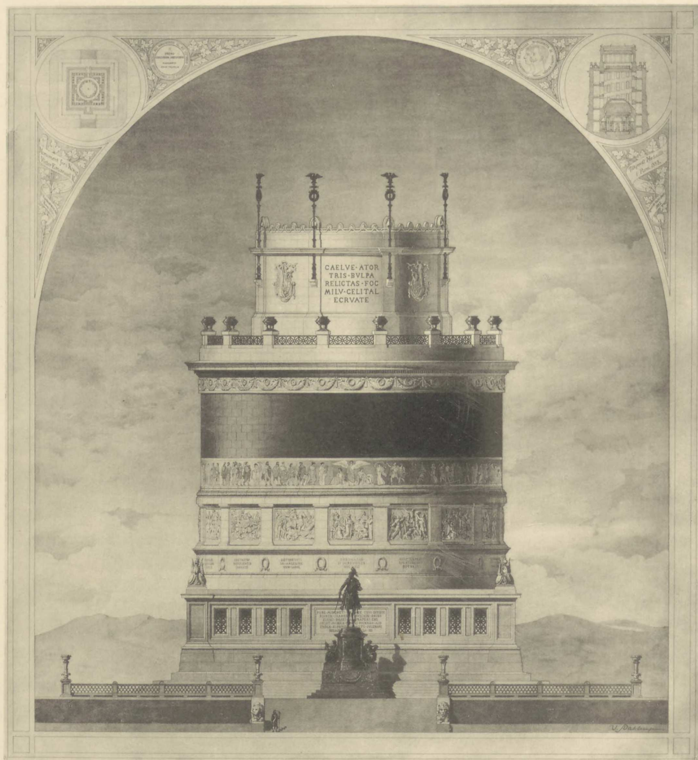
PRÆMIERET KONKURRENCE-PROJEKT TIL ET MINDESMÆRKE FOR VICTOR EMANUEL I ROM
