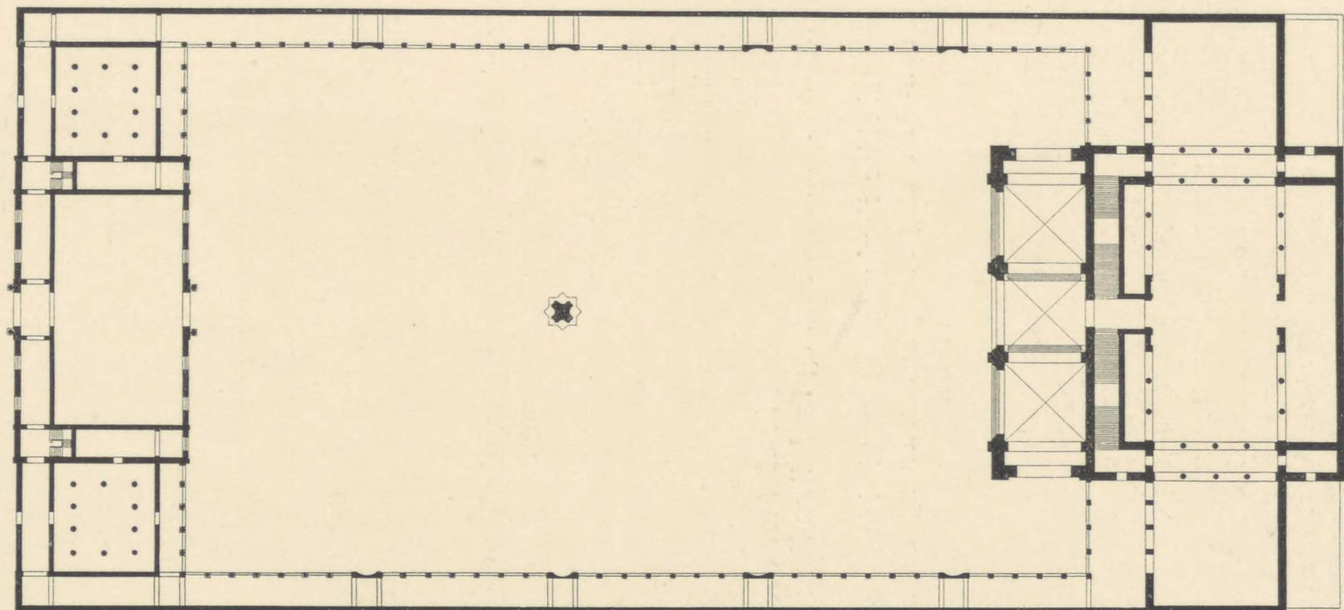
Tidligt Projekt til en Sportsplads i Ørstedsparken. Efter V. Dahlerups Tegninger.
