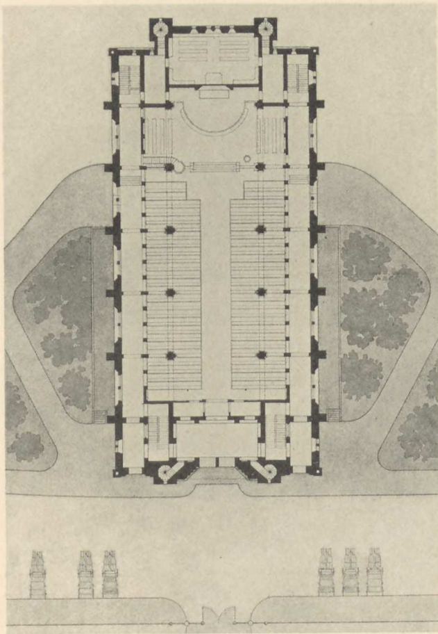
Projekt til en Kirke. Udarbejdet for den Bygge- plads, hvor Dahlerup senere opførte Søvavillonen. Efter V. Dahlerups Tegninger.
