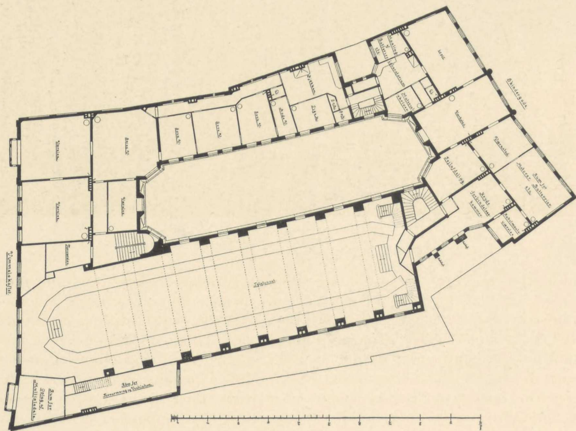
Etageplan af Bygningsanlægget i Jorcks Passage.
