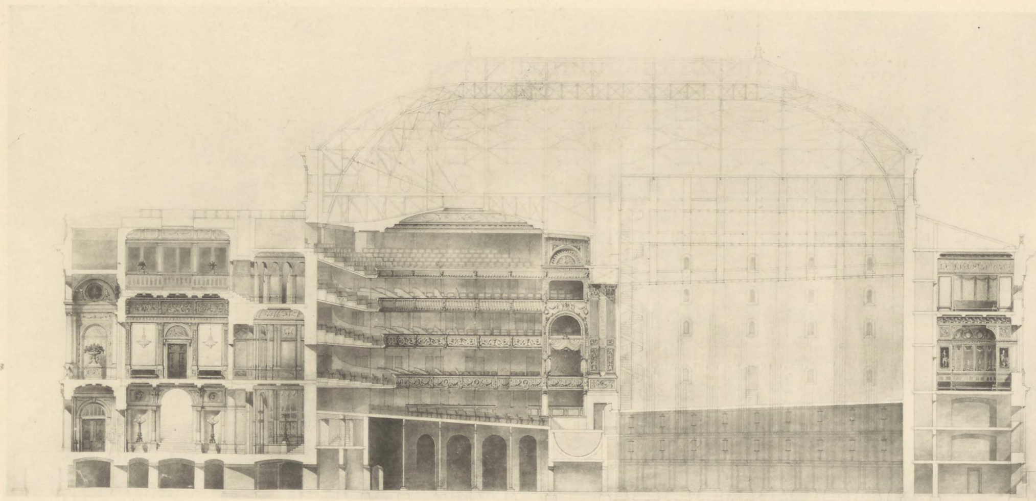
DET KGL. THEATER. LÆNGDESNIT FRA KONKURRENCEPROJEKTET Efter V. Dahlerups Tegning.
