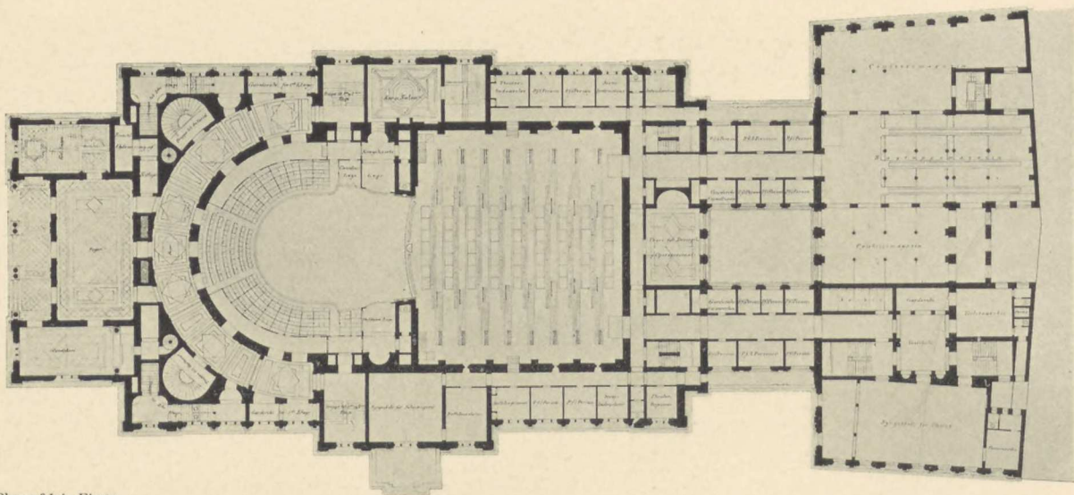
Plan af 1ste Etage.
