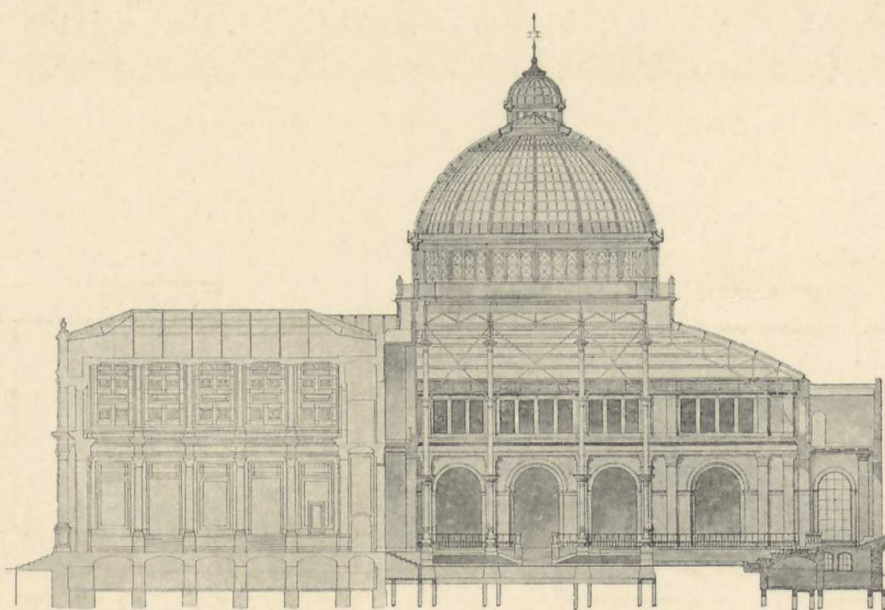
Ny Carlsberg Glyptotek med Vinterhaven. Tværsnit og Længdesnit. Efter V. Dahlerups Tegninger.
