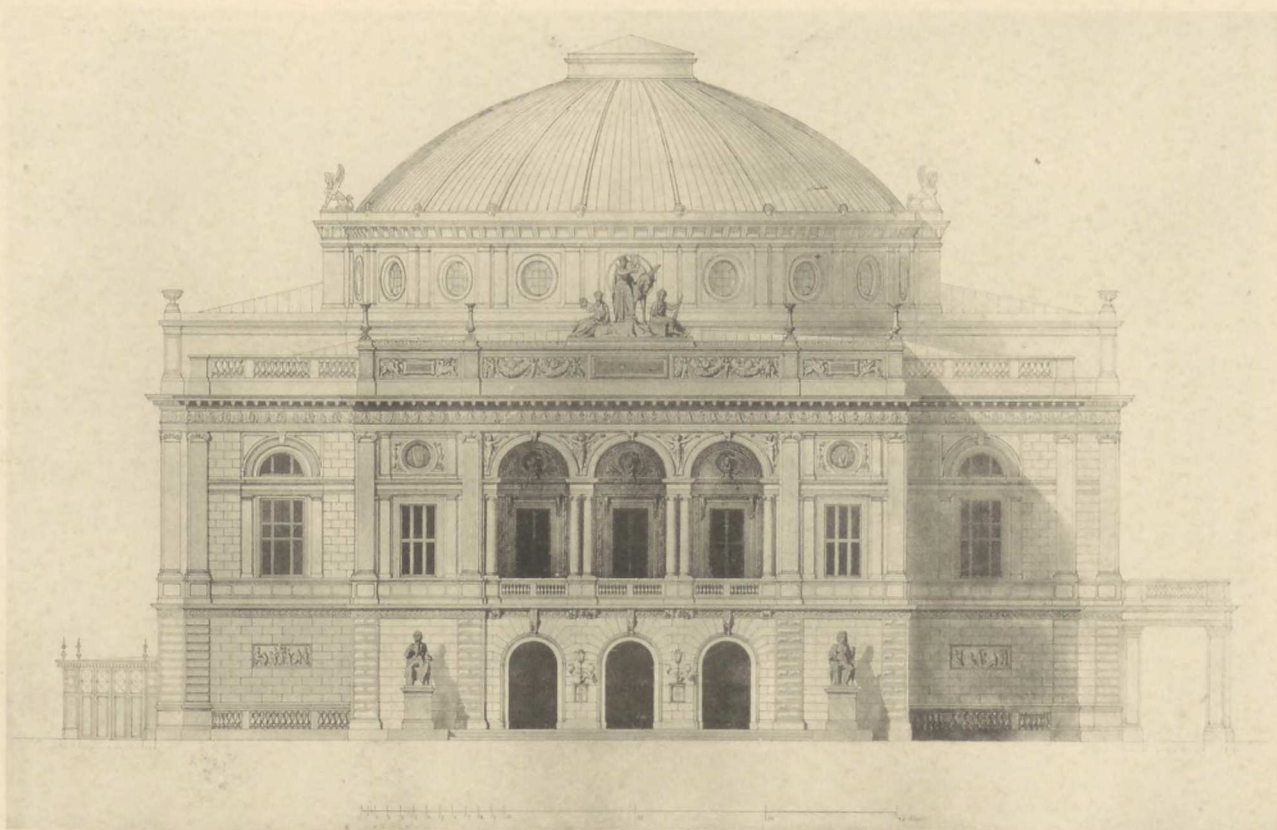
DET KGL. THEATER. FAÇADEN Efter V. Dahlerups Tegninger.
