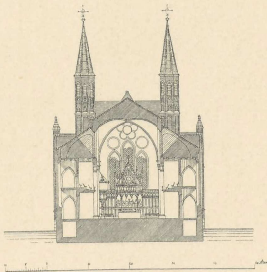
Projekt til en Kirke. Udarbejdet for den Bygge- plads, hvor Dahlerup senere opførte Søvavillonen. Efter V. Dahlerups Tegninger.
