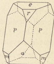
Fig. 67. Titanit. 1ste og 3die Endeflåde (a og e) Pyramide (p), Prisme (m) og Tværsdome (r).
