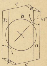
Fig. 55. Natriumthiosulfat. b 2den, c 3die Endeflade, n Prisme, p Pyramide.
