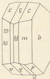
Fig. 34. Plagioklaskrystal (sml. Fig. 7) med Tvillinglameller efter b(010) .
