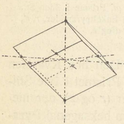
Fig. 12. Romboeder (Kalkspat).
