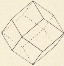
Fig. 19. Rombedodekaeder.
