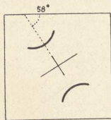
Fig. 50. Ferrocyankalium.
