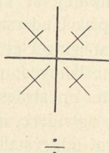
Fig. 42. Skema for en eenakset, negativ Krystal.
