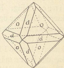
Fig. 27. Oktaeder, o, og Rombedodekaeder, d.
