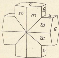
Fig. 33. Staurolit; rombisk Krystal med m(110) , c(001) og b(010) , Gennemvoksnings-tvilling efter en Langsdomeflade.
