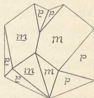
Fig. 59. Tinsten. Kombination af Prisme ( m ) og Pyramide ( p ) i 1ste Stilling; Tvilling efter en Pyramide i 2den St.
