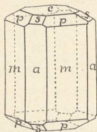
Fig. 8. Tetragonal Krystal (Vesuvian) med m (110), a (100), p (111), s (101) og c (001).
