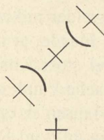
Fig. 43. Skema for en toakset, positiv Krystal.
