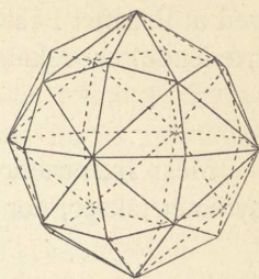
Fig. 24. Heksakisoktaeder (321).
