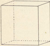
Fig. 18. Tærning.
