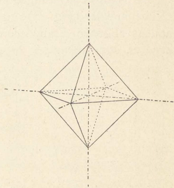
Fig. 21. Oktaeder.
