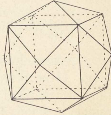
Fig. 20 Pyramidetærning (210).
