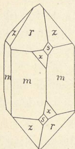
Fig. 16. Kvartskrystal („Højrekvarts“).
