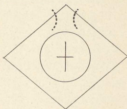
Fig. 51. Kaliumklorat.
