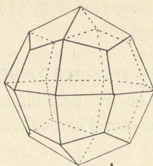
Fig. 23. Ikositetraeder (211).
