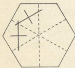
Fig. 48. Kaliumbisulfat.
