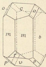
Fig. 5. Monoklin Krystal (Ortoklas) med m (110), b (010), c (001), o (021), r (201), v (101) og p (111).
