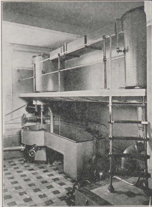
Pumpe- og Turbineanlæg.
