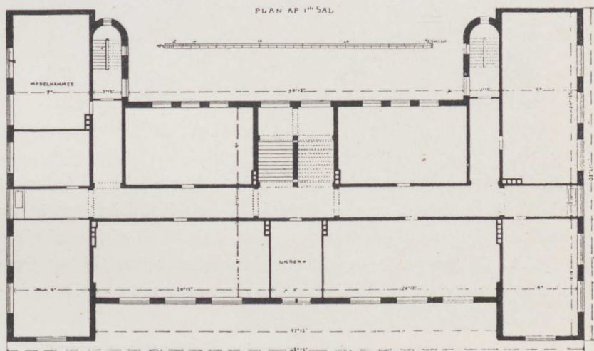
Plan af Skolens 1ste Sal.
