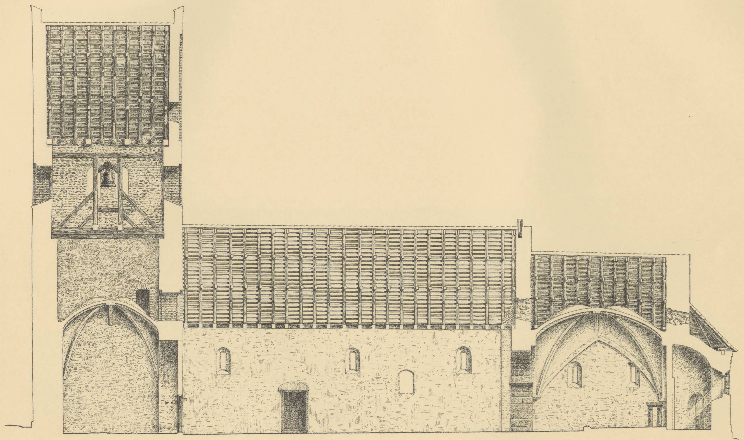
LÆNGDESNIT.
