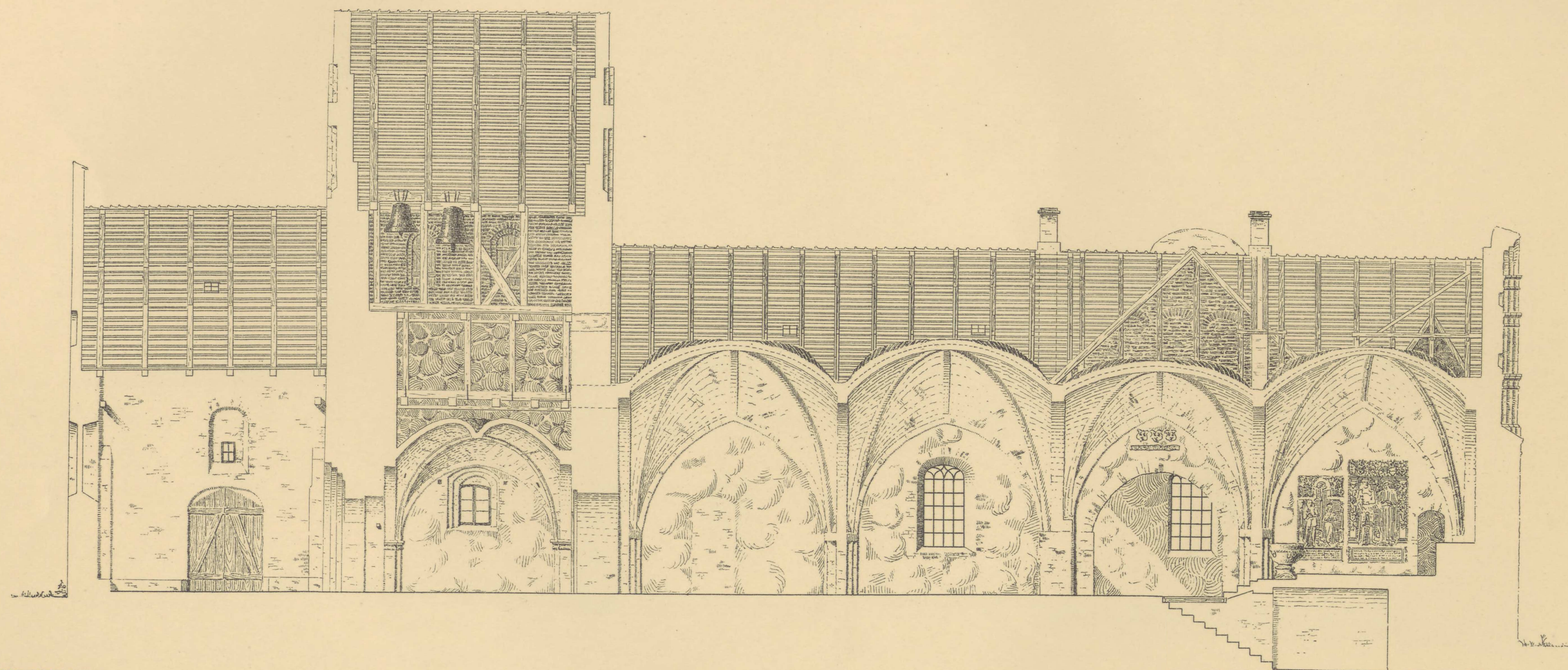
LÆNGDESnit.
