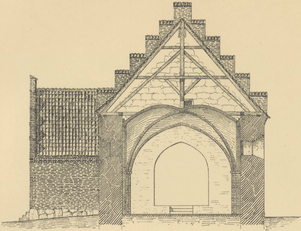
SNIT GENNEM SKIB, SET MOD ØST.
