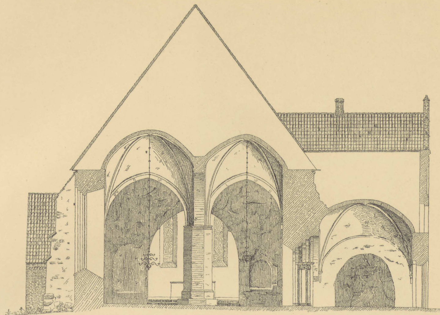
SNIT GENNEM SKIB, SET MOD ØST.
