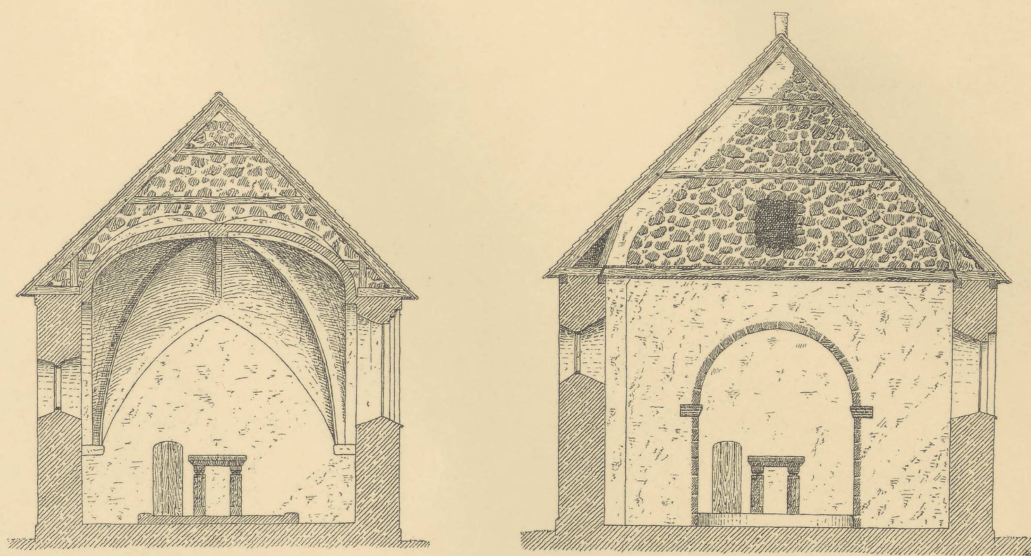
SNIT GENNEM KOR, SET MOD ØST.
