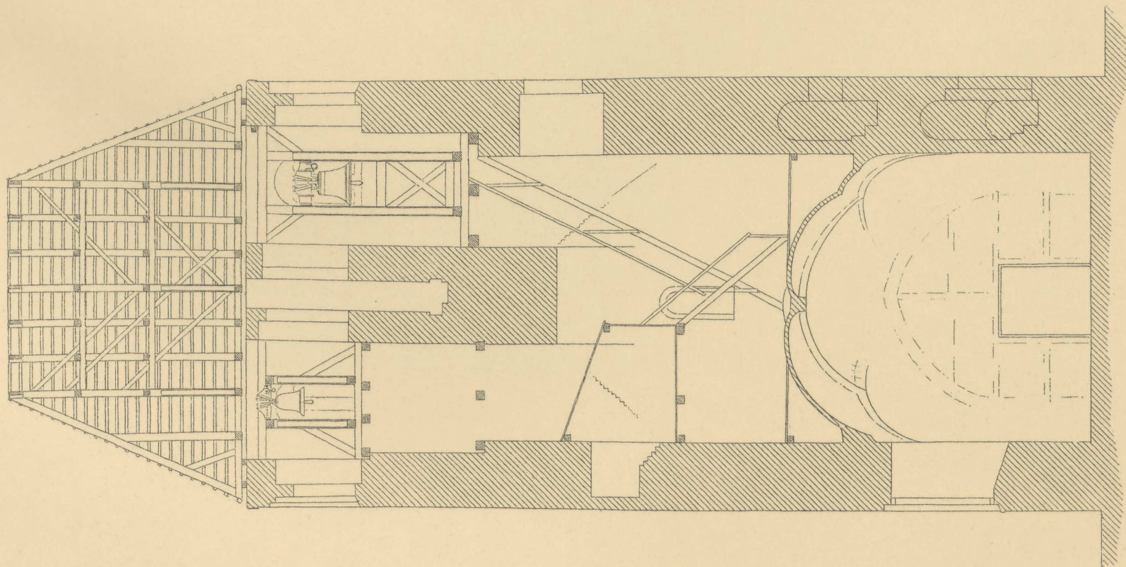
SNIT GENNEM TAARN.
