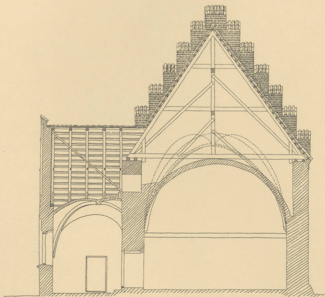
SNIT GENNEM KOR, SET MOD ØST.
