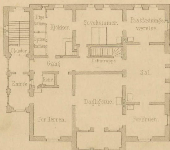
1 ste ETAGE
