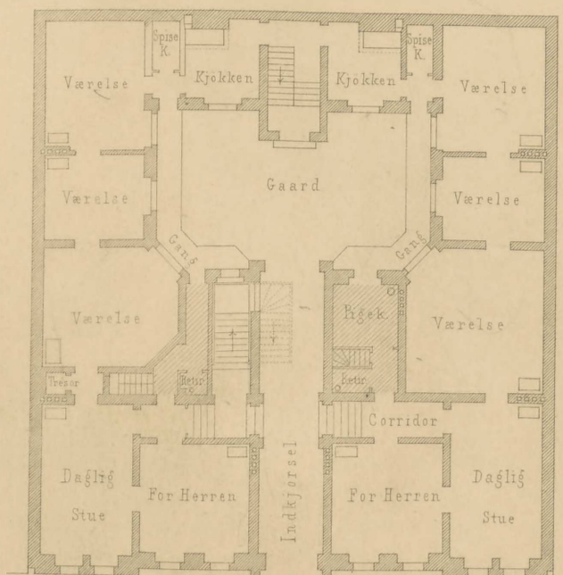
STUE ETAGE.
