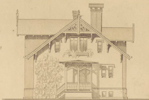
Östlige Cavl.
