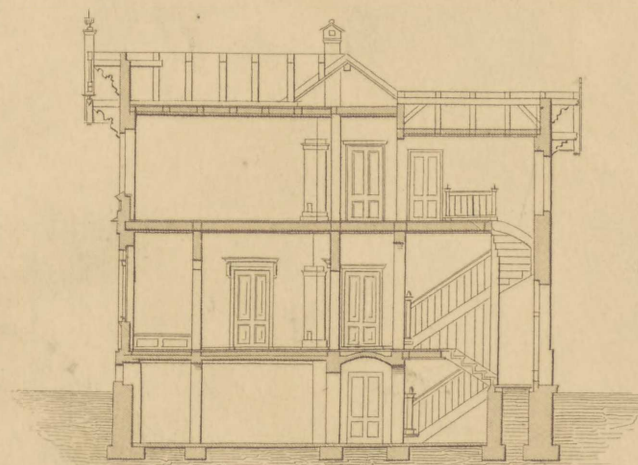
Gjennemsnit efter A.B.
