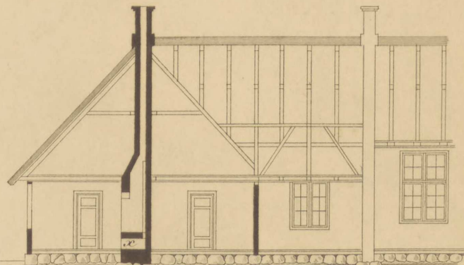
Snit efter Linien A.B.
