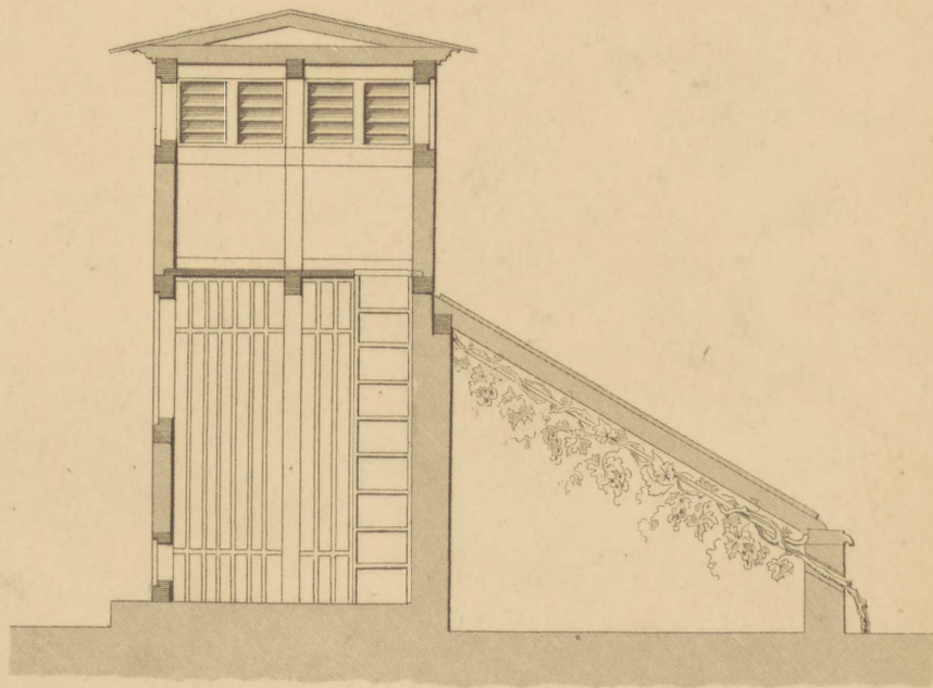
Profiler.
