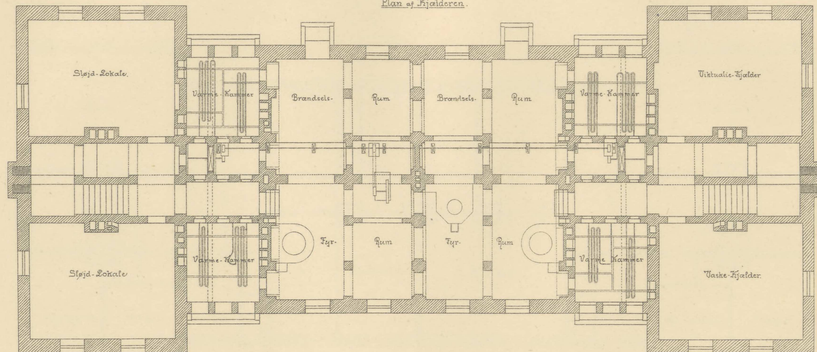
Plan af Kælderen.
