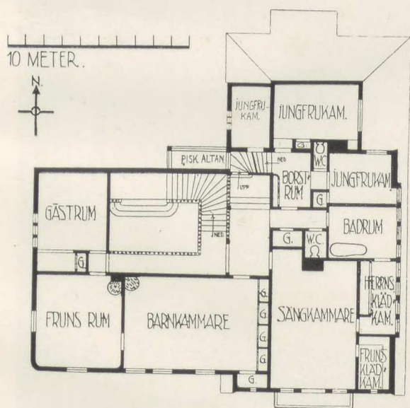
LAURINS BOSTAD. DJURGÅRDEN — VÅNINGEN 1 TR. UPP
