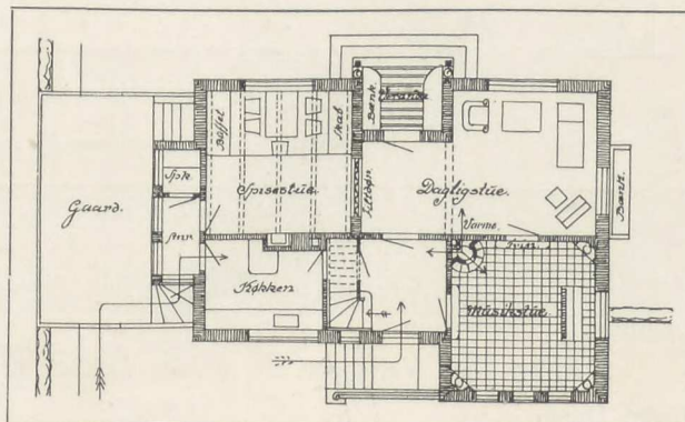
Stueplan af samme.
