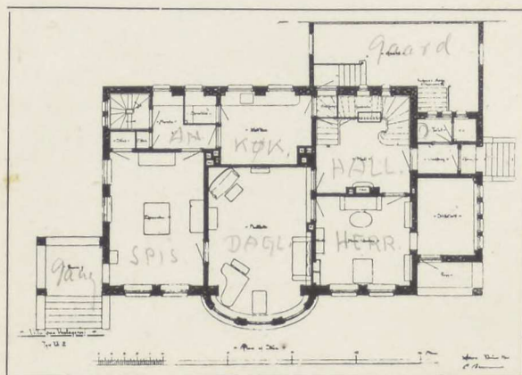
Plan af Red. Gulmanns Villa.
