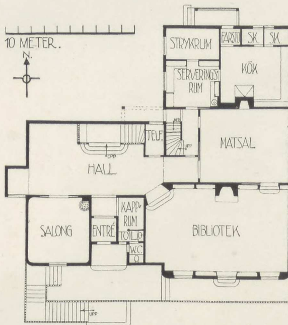
LAURINS BOSTAD. DJURGÅRDEN — BOTTENVÅNINGEN
