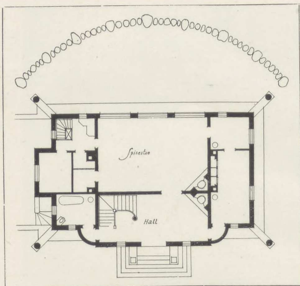
Plan til Kalø Jagthus.
