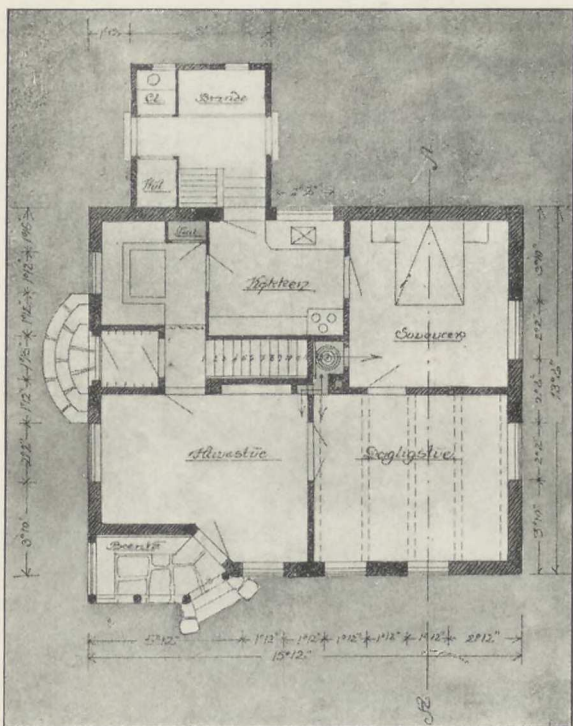
Plan af ovenstaaende.
