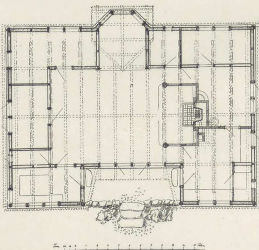
Plan af samme.
