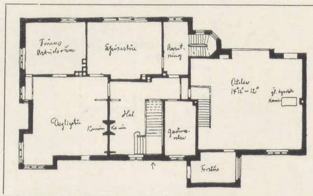
Stueplan af ovenstaaende Hus.
