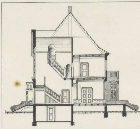
Tværsnit af samme Villa.
