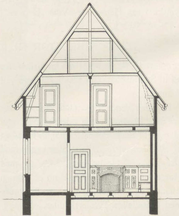
Snit af samme.
