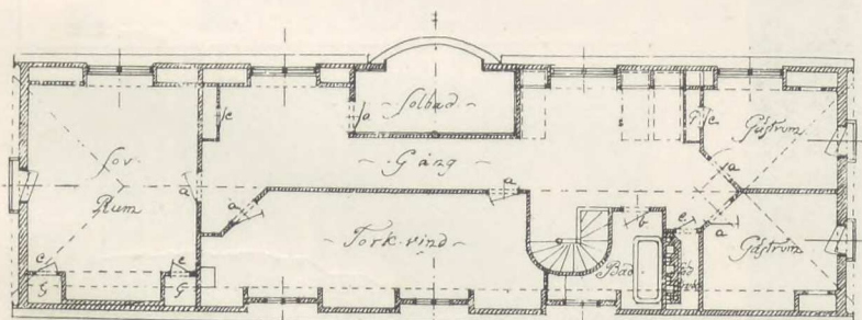
Plan af første Sal.
