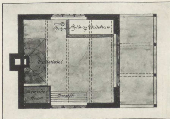
Vaske-, Bade- og Lysthus til en Villa ved Aarhus.
