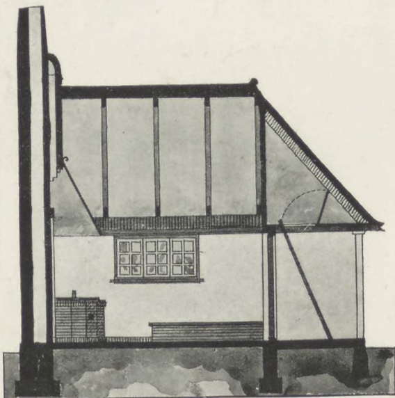
Vaske-, Bade- og Lysthus til en Villa ved Aarhus.
