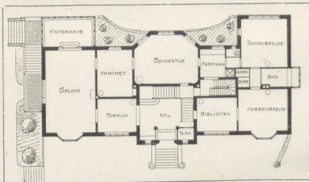
Plan af Villa „Bernina“.
