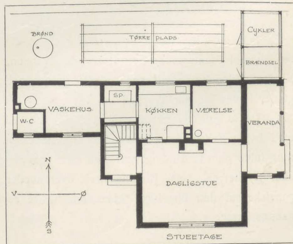
Plan af eget Hus.
