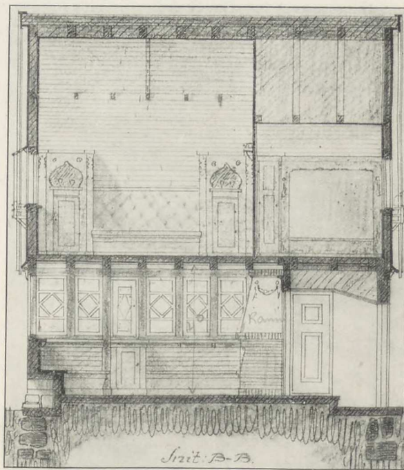
PLAN OG SNIT AF OVENSTAAENDE BILLIGE SOMMERHUS
