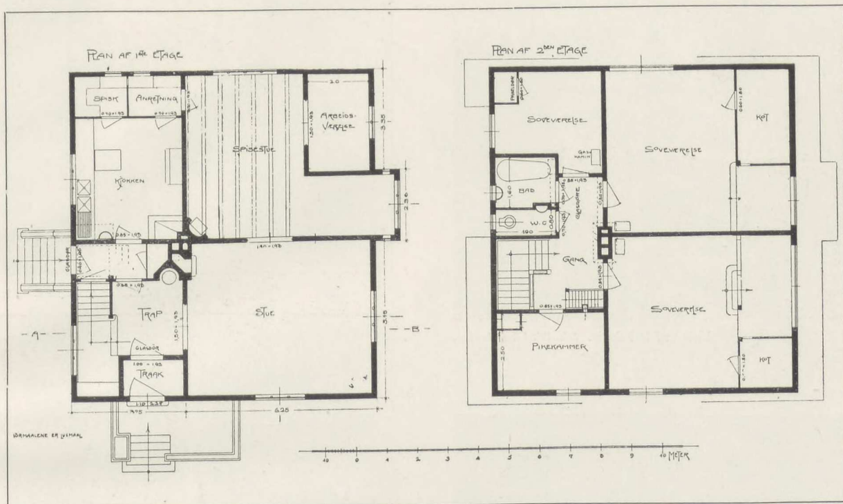
Planer af Prof. Bugge's eget Hus. (Side 52.)
