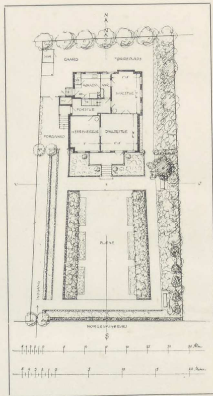
Plan af samme.
