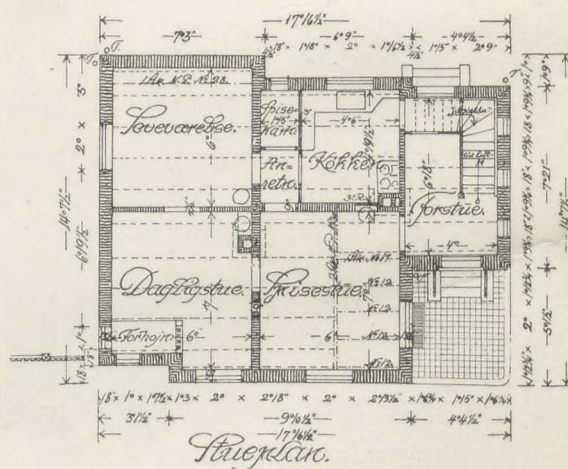
Portnerboligen ved Fyns Stifts Sparekasse i Odense.
