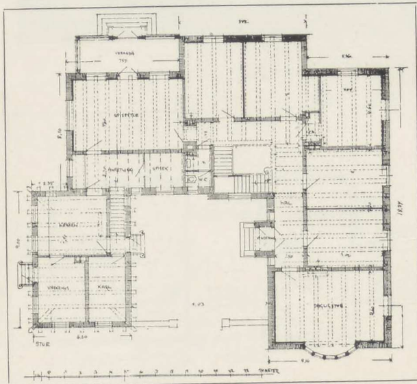
Plan af „Th. Wessels Minde“.
