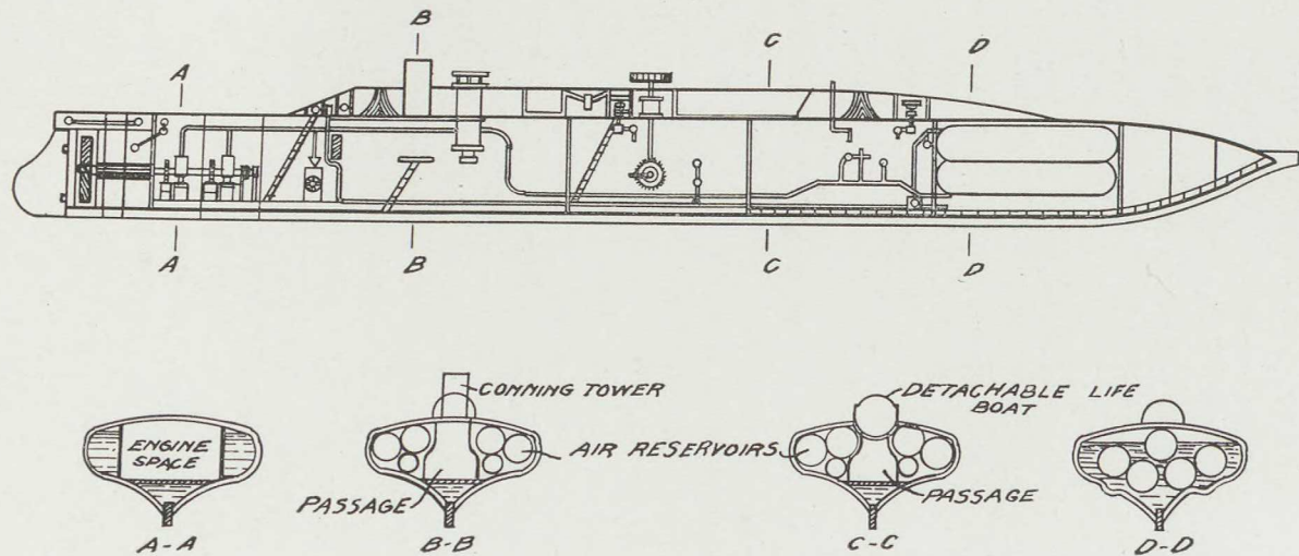
Le Plongeur. 1863
