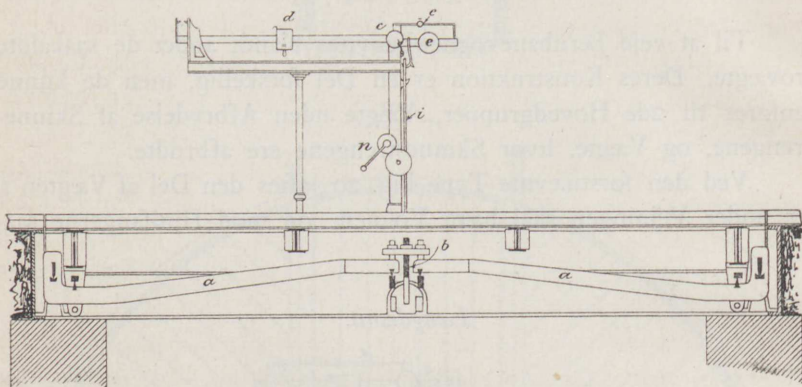
Tværsnit.
