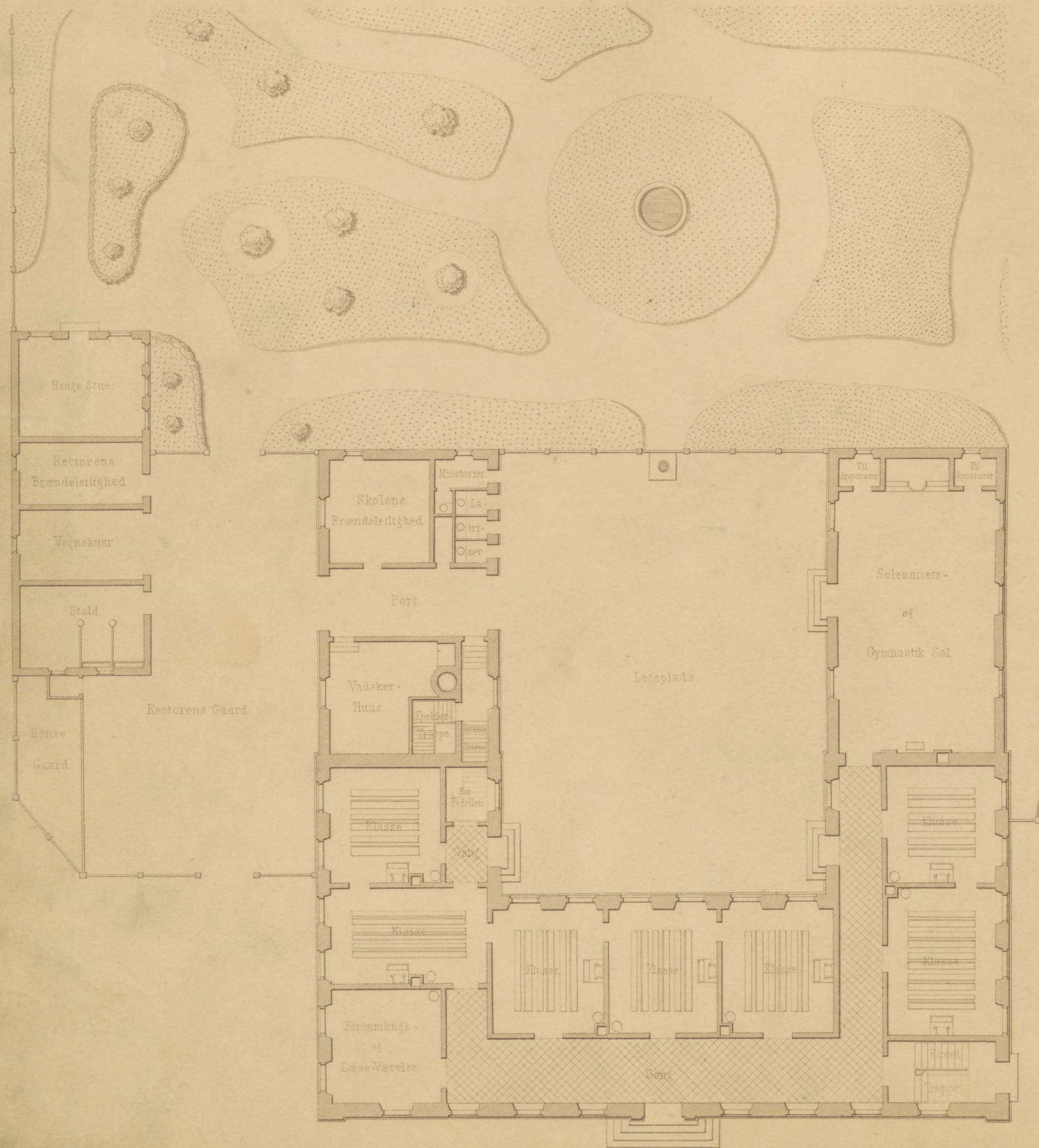
Plan af 1 ste Etage (Stuen.)
