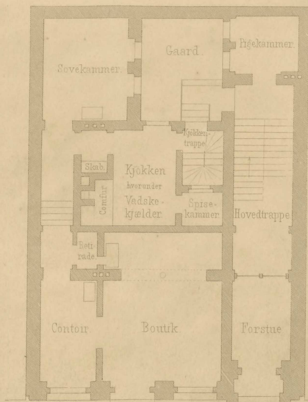
Plan af Stuen.
