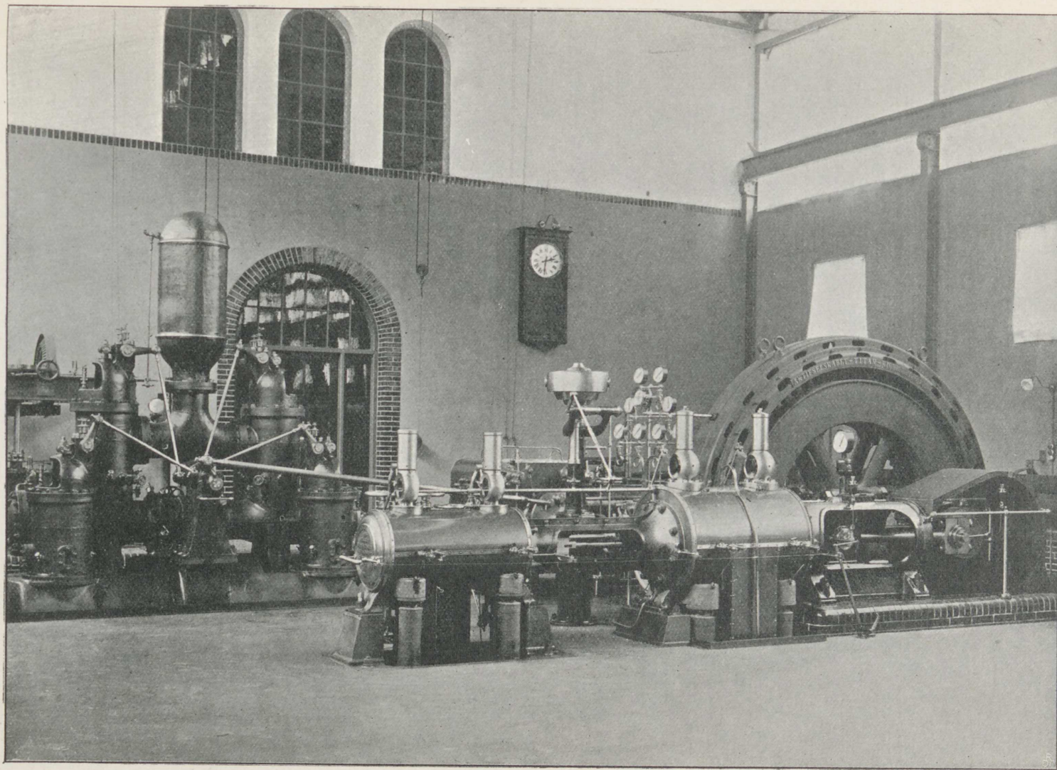
Fig. 36. Hoveddampmaskinen.
