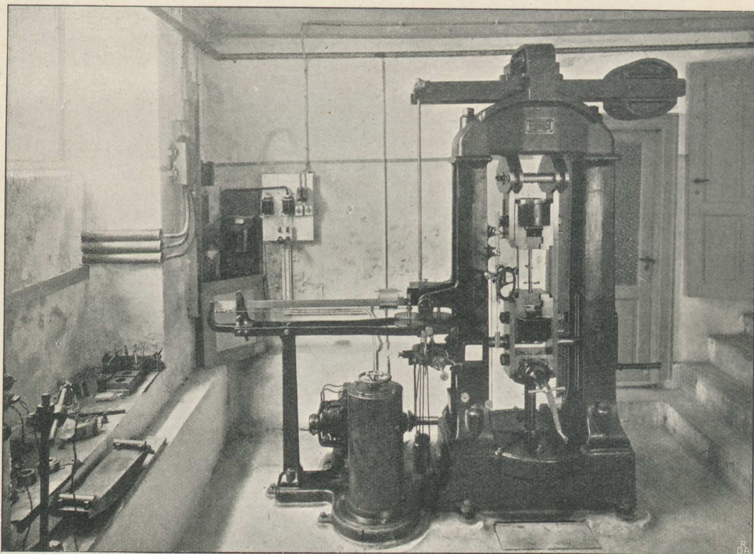
Fig. 68. Universalprøvemaskine.
