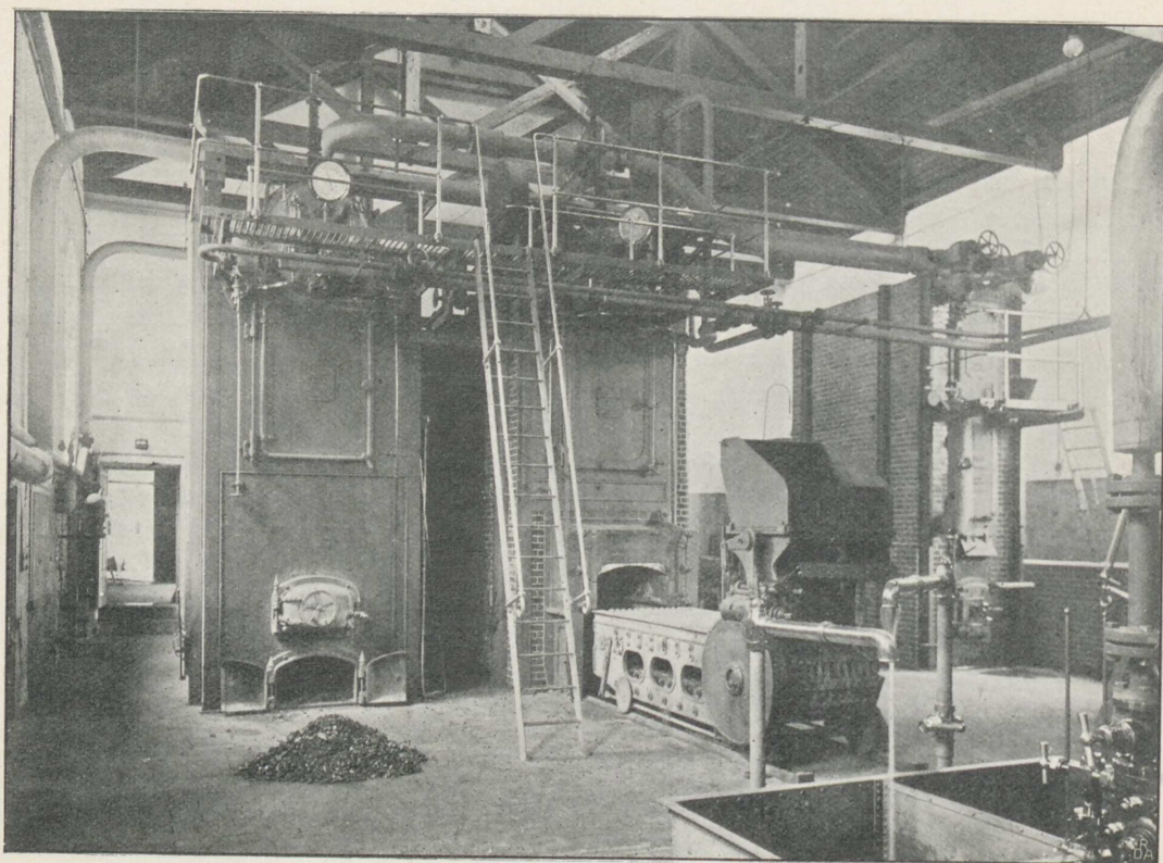
Fig. 40. Kedelanlæg.
