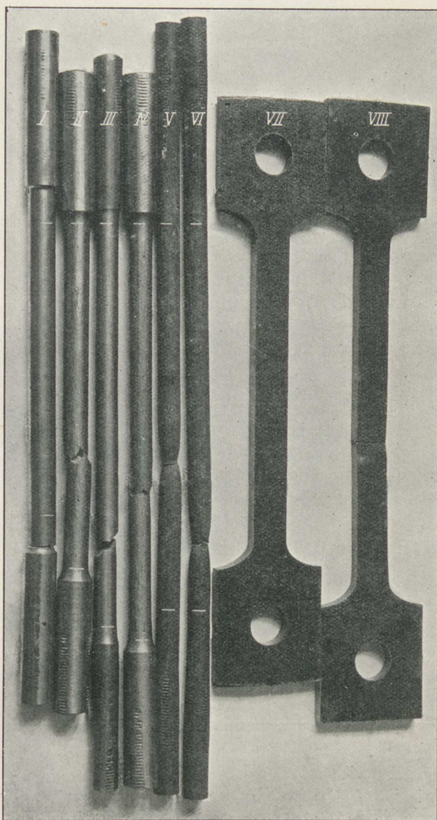
Fig. 64. Strækprøver.
