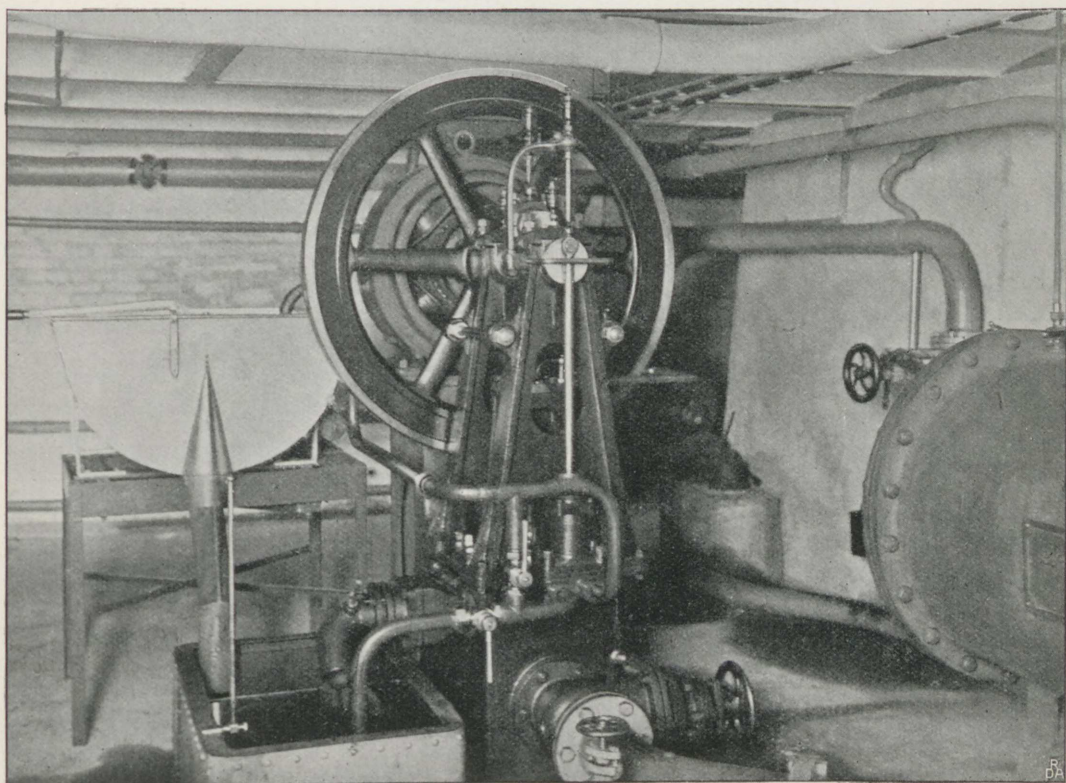
Fig. 38. Kondensationsanlæg.
