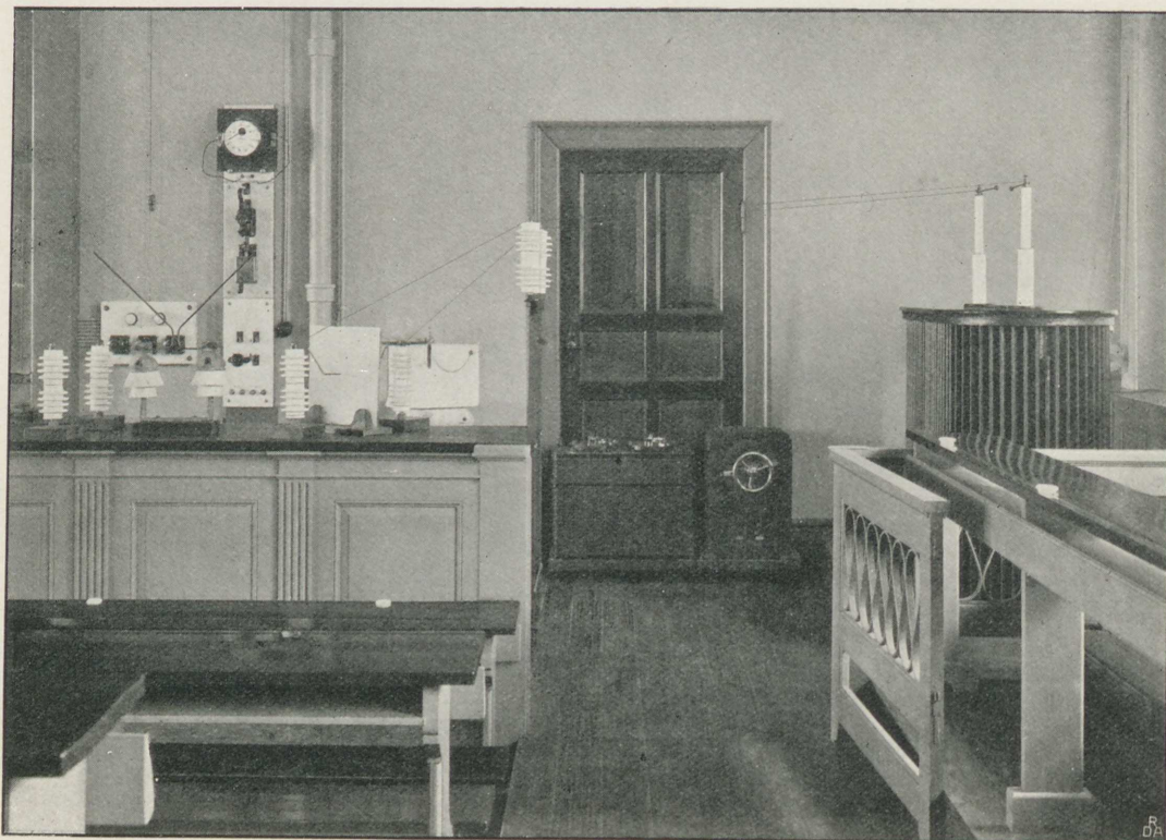
Fig. 62. Transformator til 100,000 Volt i det elektrotekniske Auditorium.
