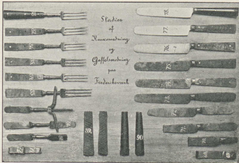
Fig. 44. Fabrikationsstadier af Bordknive og -gaffer.
