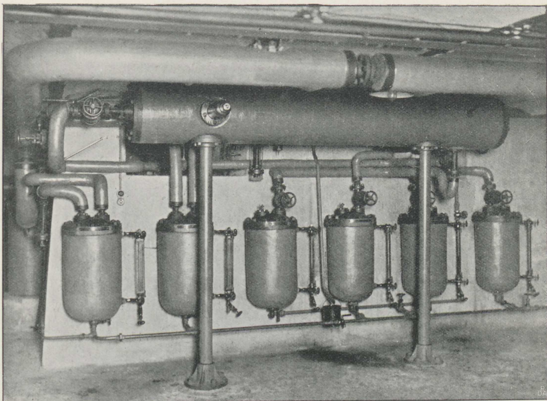
Fig. 37. Vandsamlere for Hoveddampmaskinen.
