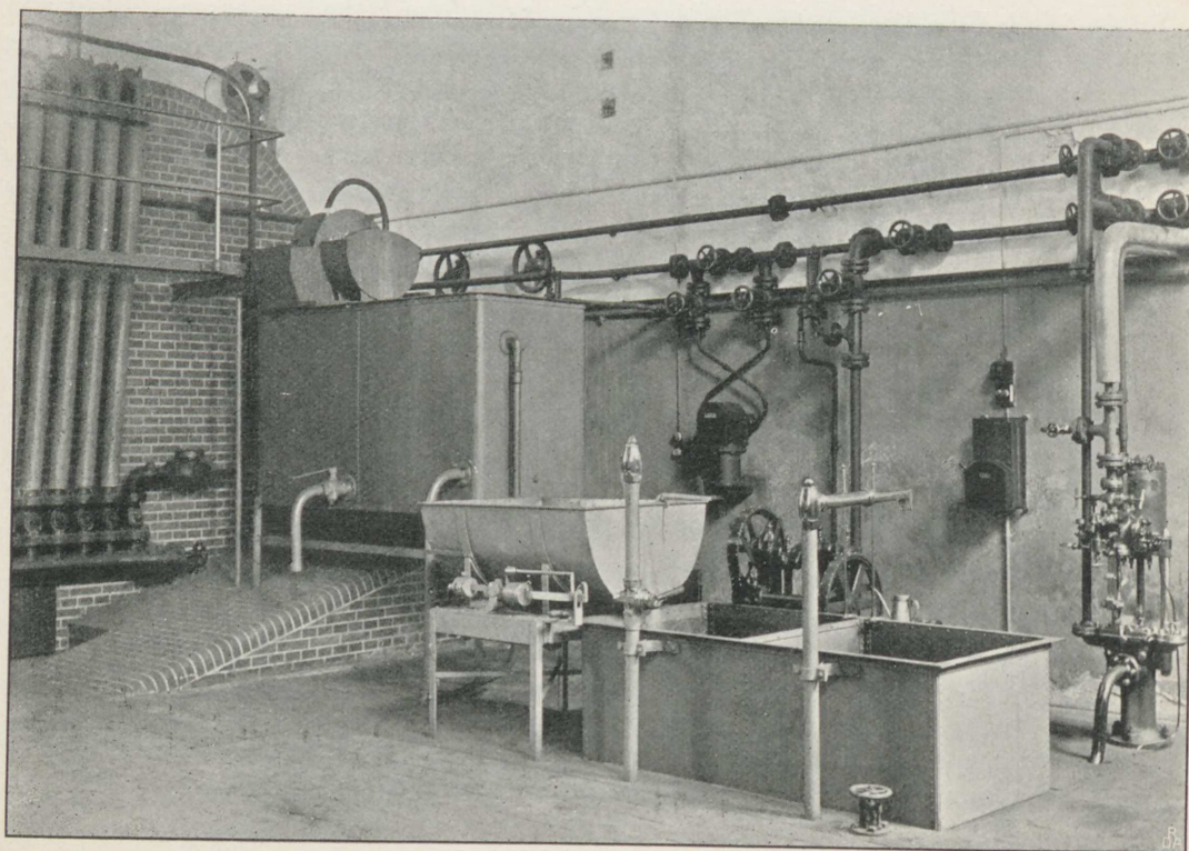
Fig. 41. Fødepumpearrangement.
