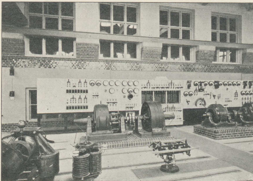
Fig. 57. Maskinsal med Omformergrupper og Hovedstrømtavle.
