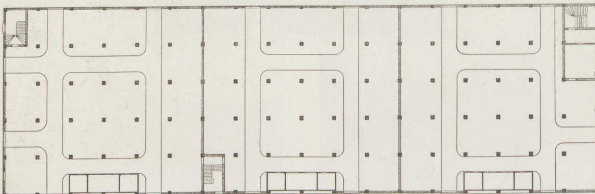
PAKHUSE I ST. PETERSBORG HAVN. Bygherre: DET NORDISKE DAMSKIBSSELSKAB, ST. PETERSBORG. CHRISTIANI & NIELSEN.
