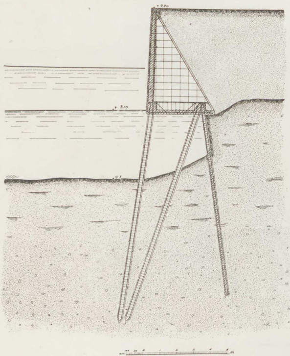
UDVIDELSE AF HAMBORG HAVN. 400 lbm. Kaimur ved Rosskanal, Neuhoj.
