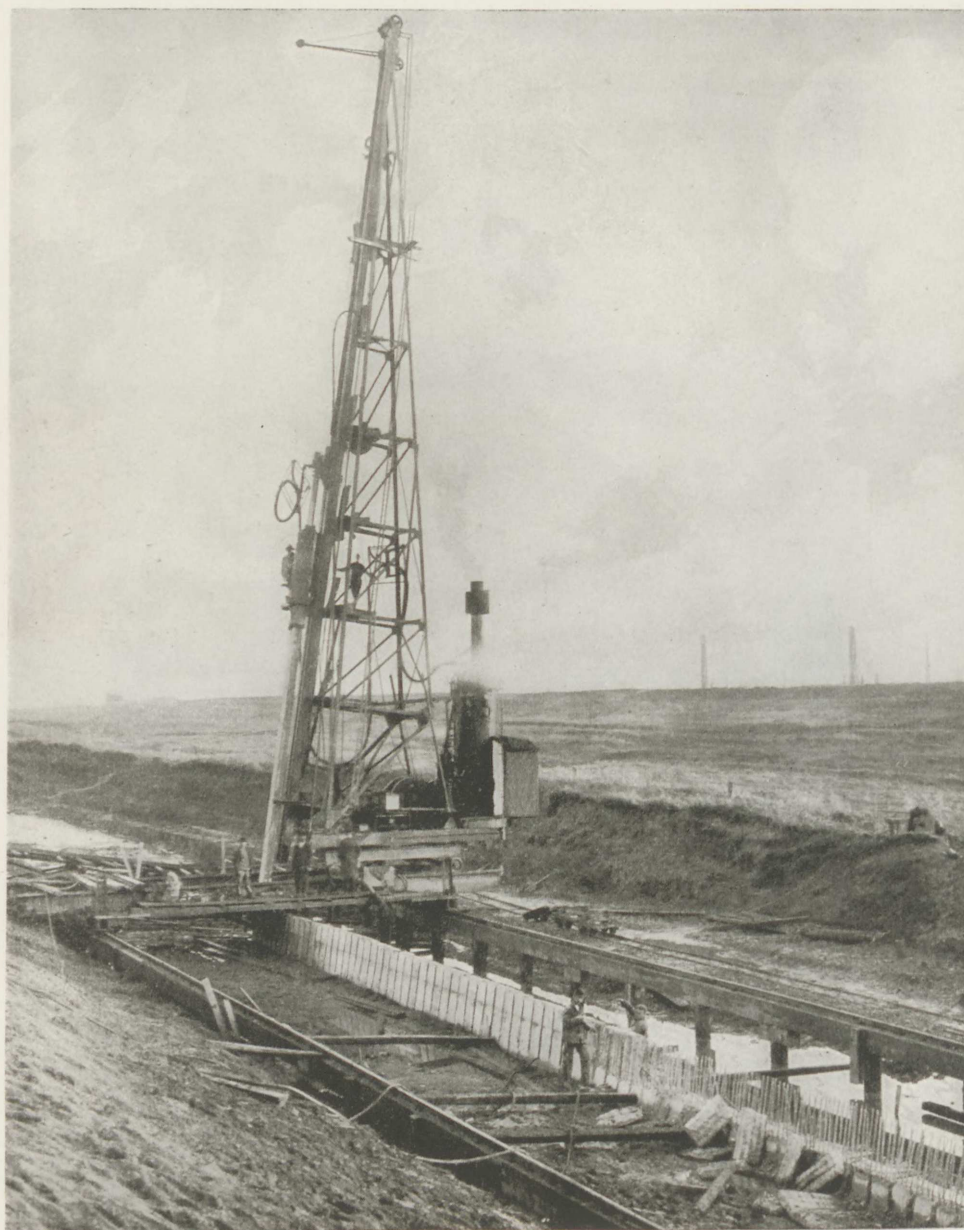
RAMNING AF JERNBETONSPUNSVÆGGE ved Udvidelsen af Hamborg Havn.
