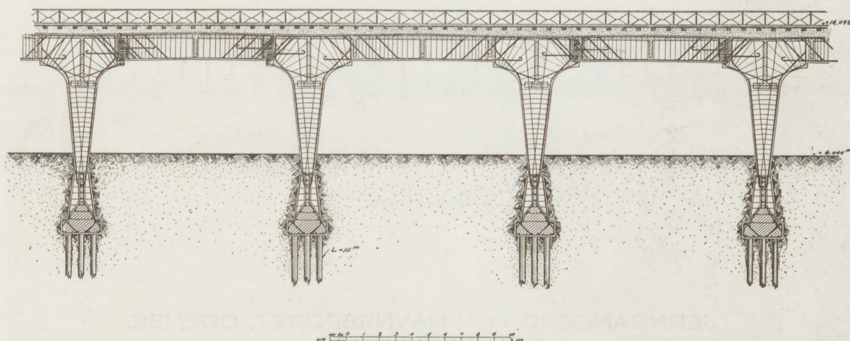
Længdesnit.
