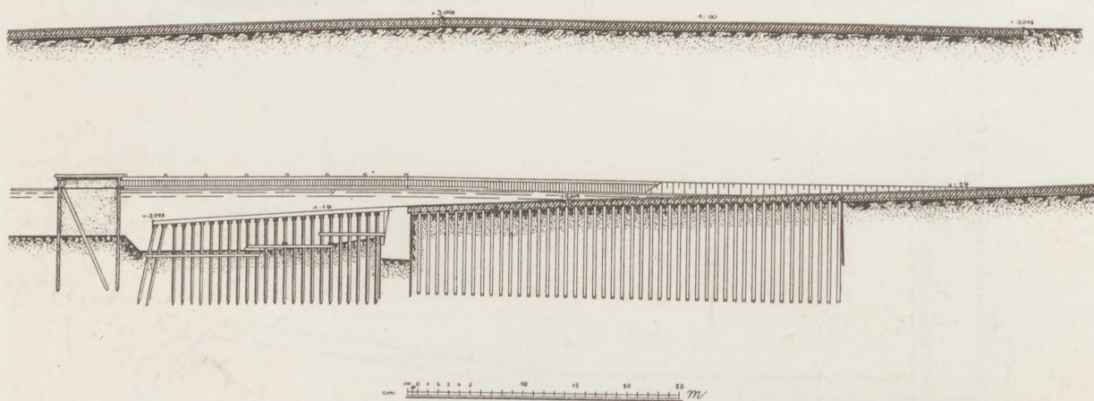
Længdesnit.
