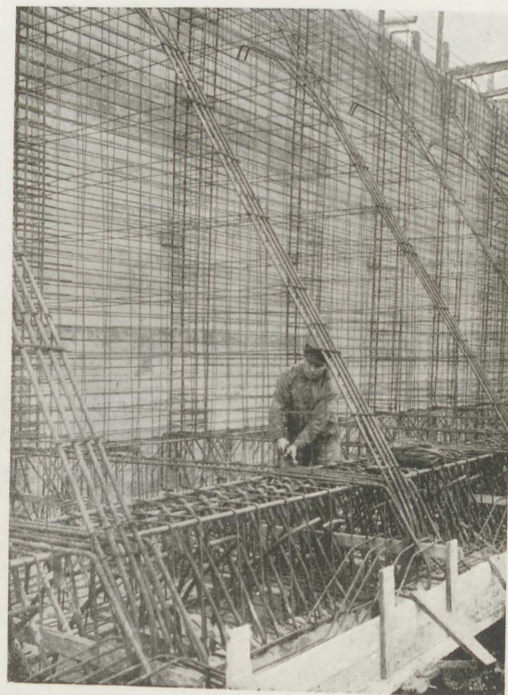
UDVIDELSE AF HAMBORG HAVN. 400 lbm. Kaimur ved Rosskanal, Neuhoj.
