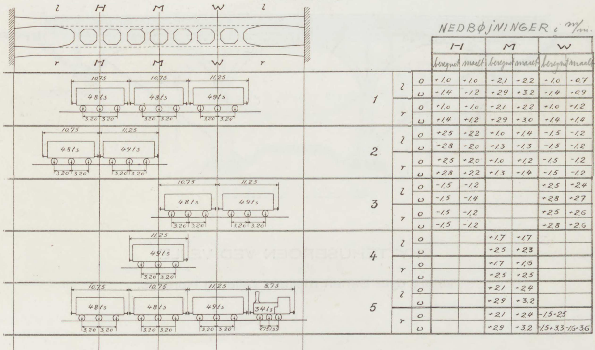
Prøvebelastning.
