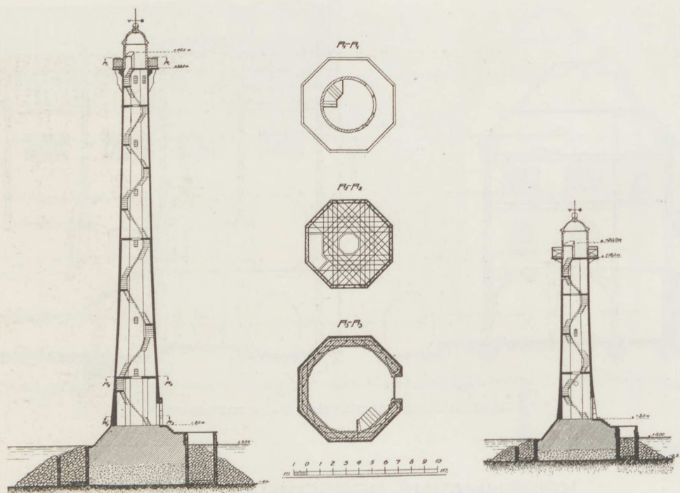
FYRTAARNE VED SØKANALEN ST. PETERSBORG-KRONSTADT.
