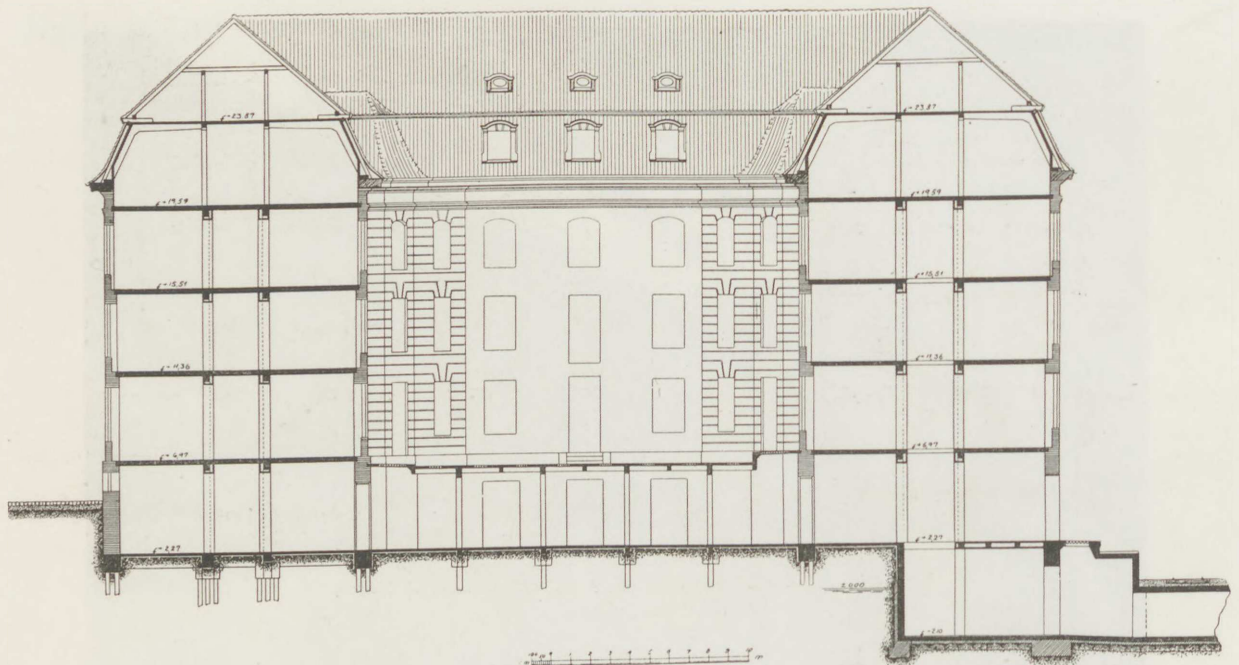
CENTRALPOSTBYGNINGEN I KØBENHAVN.
