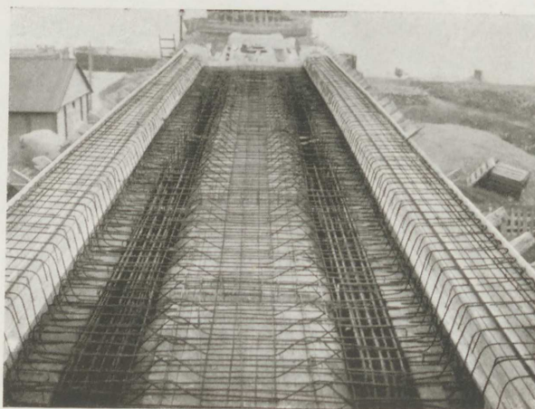
JERNBANE BRO I ST. PETERSBORG 600 Meter Længde.
