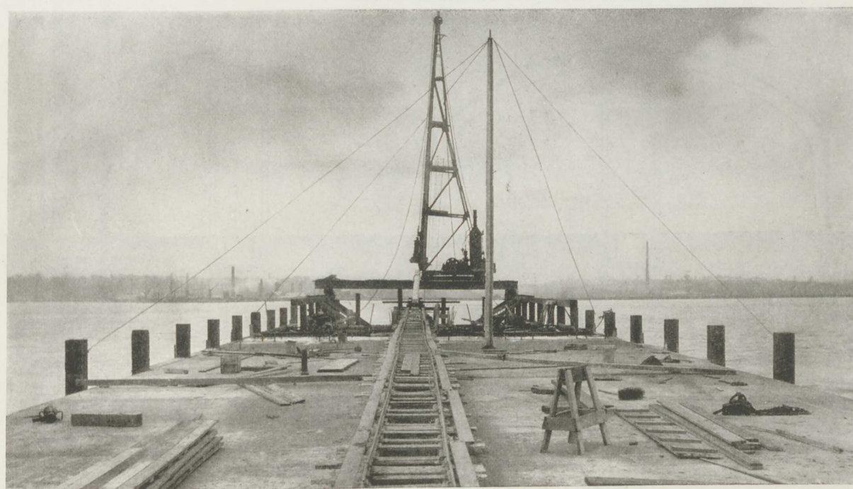
PIERANLÆG VED THEMSEN I GRAYS, LONDON
