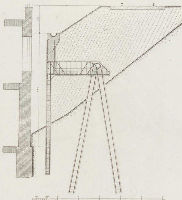
STØTTEMUR VED BANEGAARDEN STERNSCHANZE I HAMBORG. Bygherre: DEN KGL. JERNBANEDIREKTION I ALTONA.
