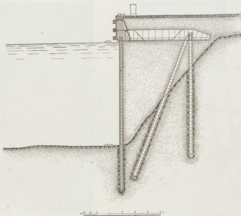
HAVNEANLÆG I HELSINGØR Kaimur, Pier og Molehoved af Jernbeton.
