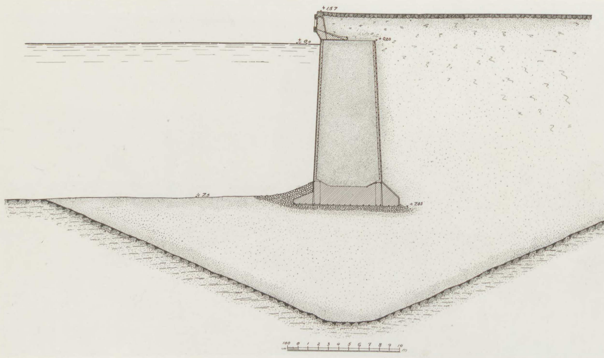
HAVNEANLÆG I NØRRESUNDBY 220 lbm. Kaimur bygget paa Sænkekasser.
